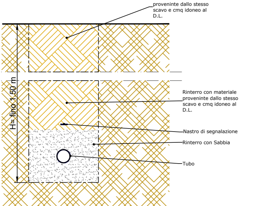
SCAVO SU TERRA FINO H.1.50 m
