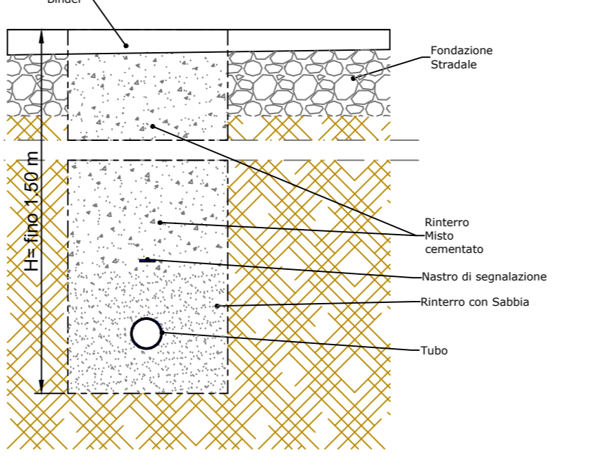
SCAVO SU STRADA FINO H.1.50 m
