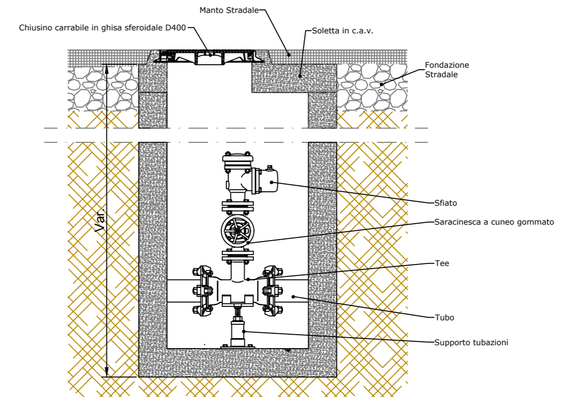
POZZETTO DI SFILATO PER ACQUEDOTTO
