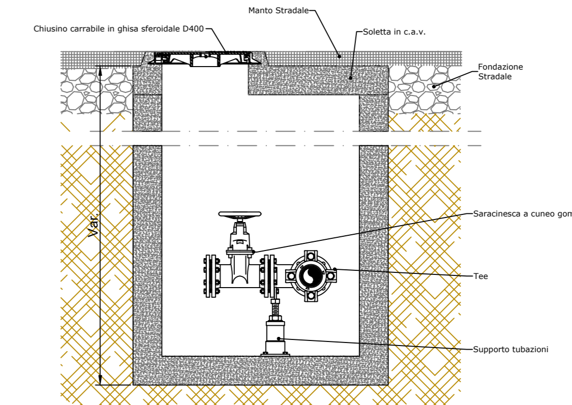
POZZETTO DI SCARICO PER ACQUEDOTTO
