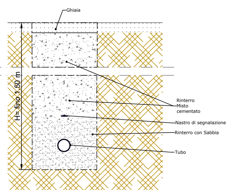
SCAVO SU GHIAIA
