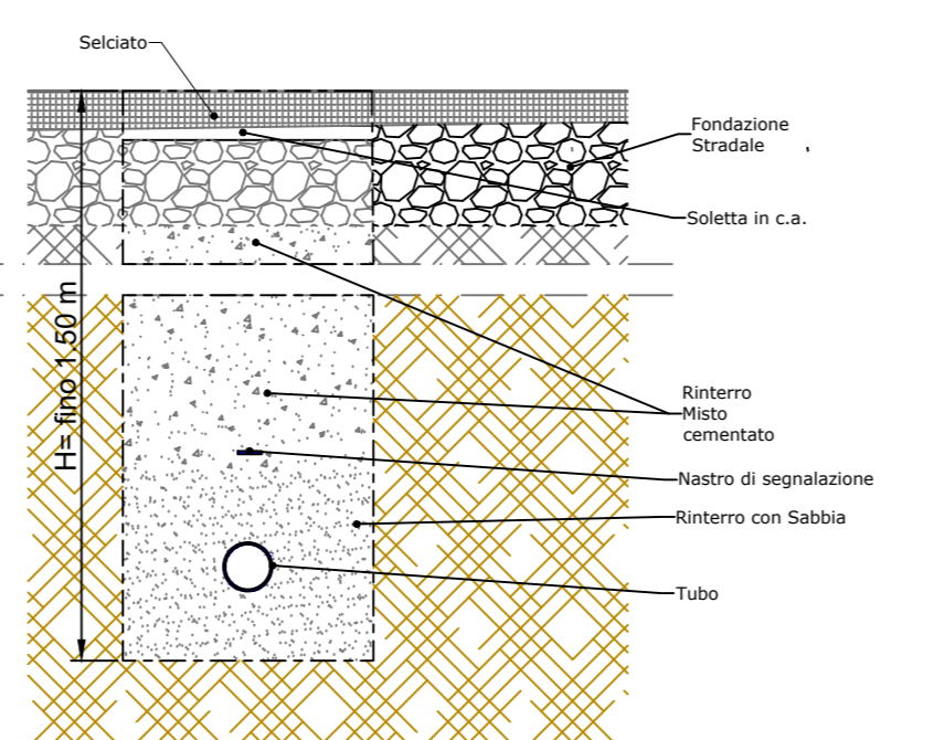
SCAVO SU SELCIATO
