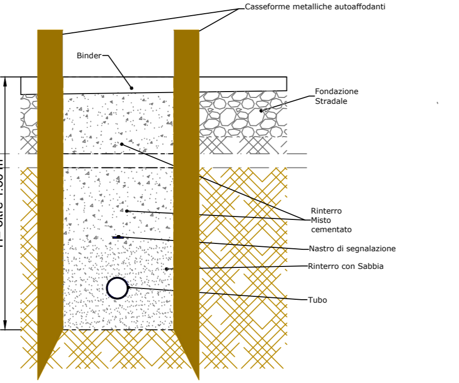
SCAVO SU STRADA OLTRE H.1.50 m
